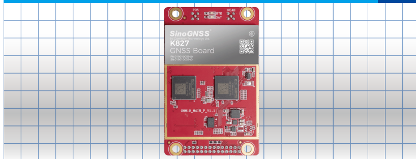
45.7mm×71.1mm×9.15mm
